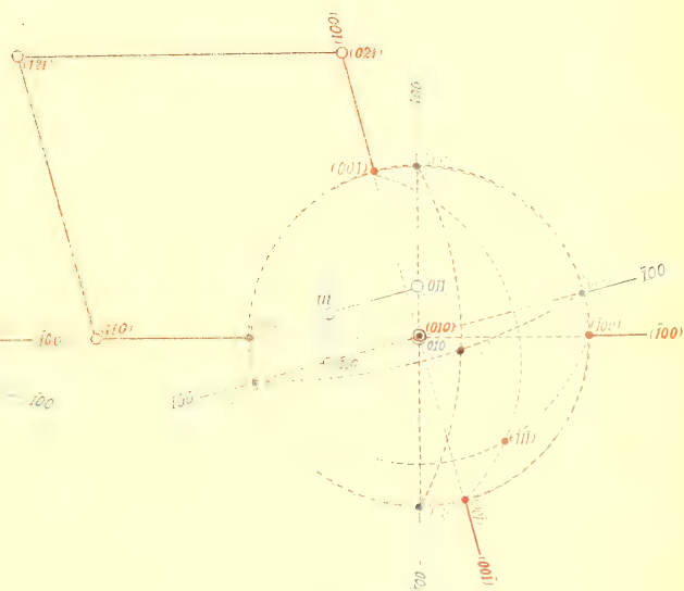
8. Аурипигмент.
